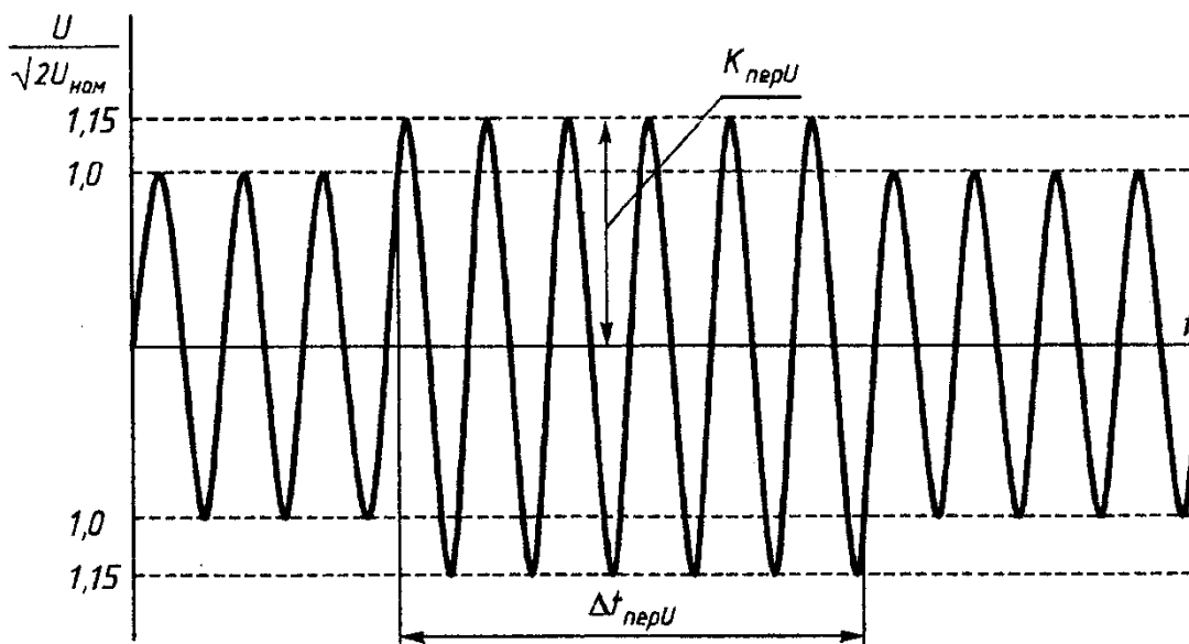
Рисунок Б.4 — Временное перенапряжение
