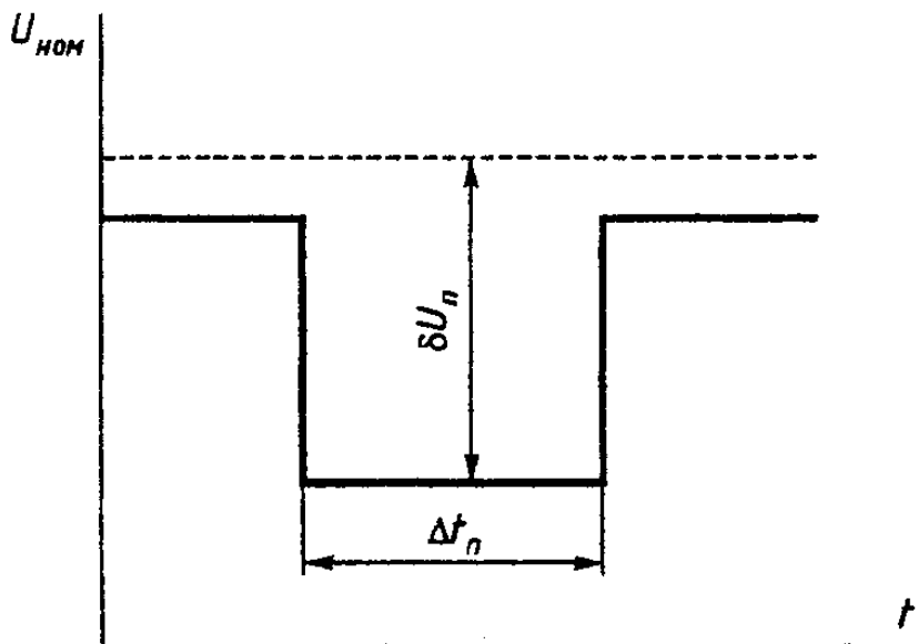
Рисунок Б.2 — Провал напряжения
