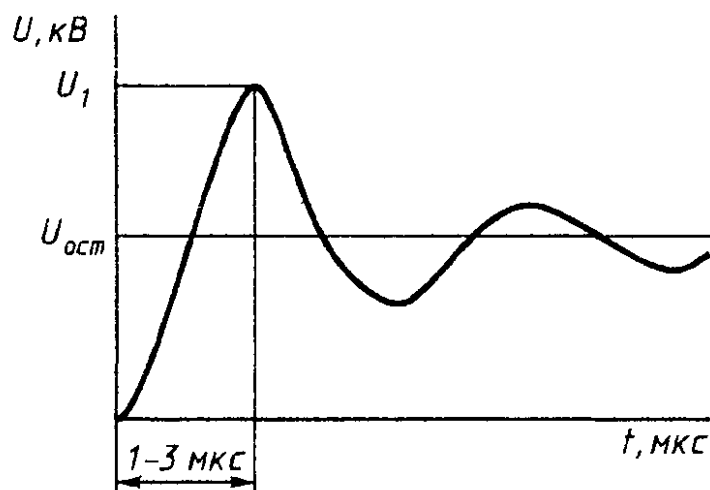
Рисунок Д.2 — Форма грозových импульсов, характерная для точек присоединения a , b , г , д на рисунке Д.1.
