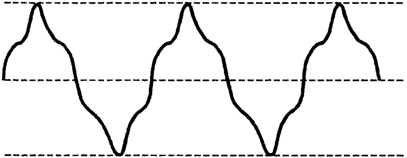
"Рис. А.1 Отклонение, колебание и провал напряжения"
