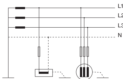
Сеть TT
